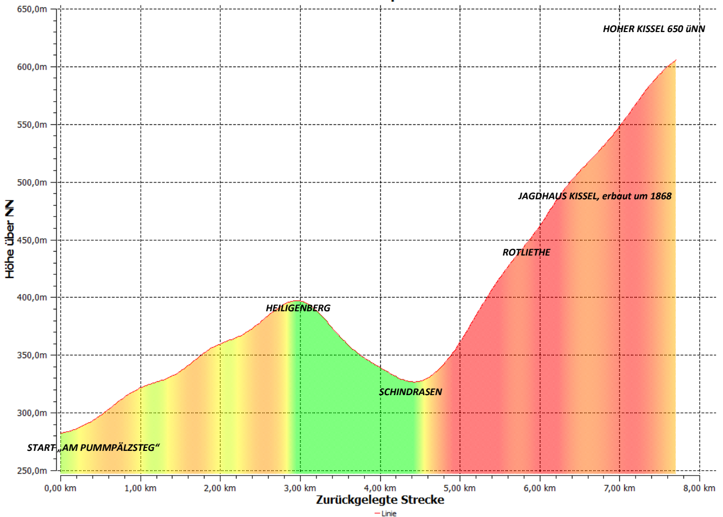
Höhenprofil
